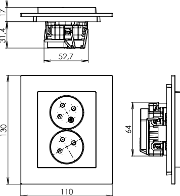
zásuvka dvojnásobná s clonkou a přepětovou ochranou (zvuková a světelná signalizace)
