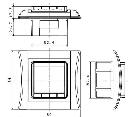
digitální termostat DSE 4T
