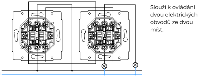
spínač řazení 6+6 dvojitý schodišťový vypínač (střídavý přepínač)
