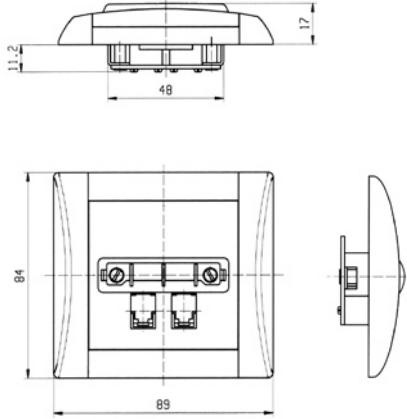
zásuvka telefonní
