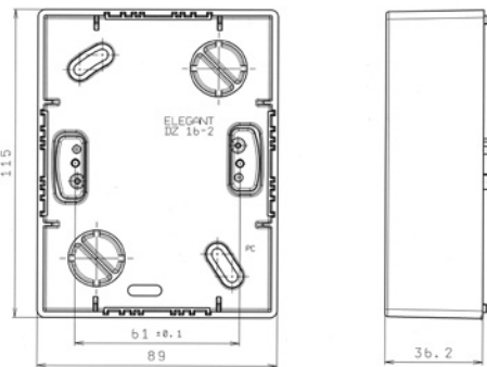
elektroinstalační krabice pro lištové rozvody pro dvojzásuvku
