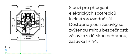
zásuvka jednonásobná
