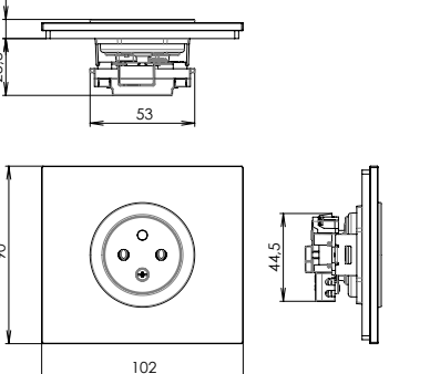
zásuvka jednonásobná s dětskou clonkou
