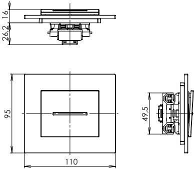
spínač s jednoduchým krytem a prosvětlením
