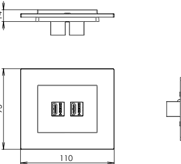
zásuvka konektorová modulová HDMI, USB, RJ 45 ...
