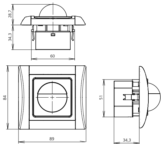
pohybové čidlo B.E.G.
