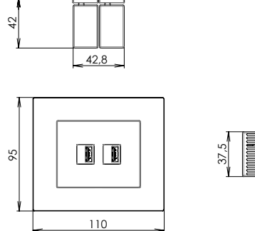
zásuvka modulová USB nabíječka
