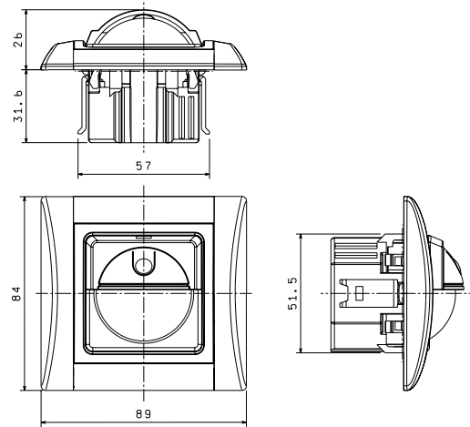
pohybové čidlo STEINEL
