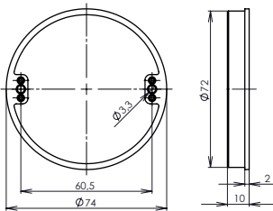
vymezovací kroužek VK1
