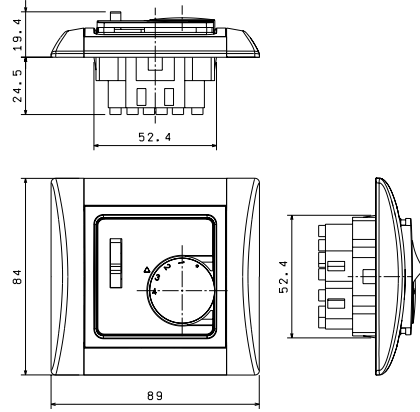
analogový termostat OREG/EBERLE DSE 2T/3T
