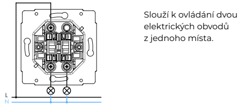
spínač řazení 5 (sériový přepínač, jednopolový přepínač dvou obvodů s polohou vypnuto)
