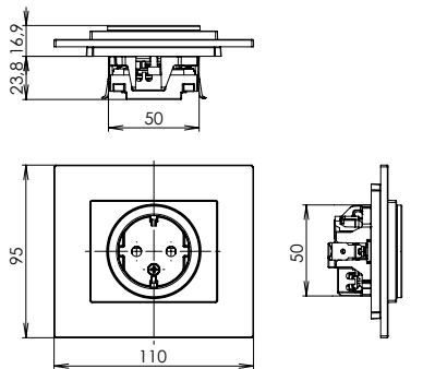
zásuvka jednonásobná schuko s clonkou
