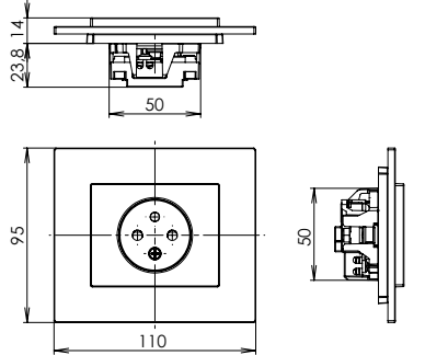
zásuvka jednonásobná s clonkou
