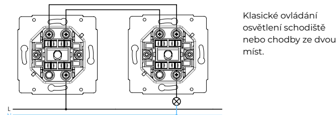
spínač řazení 6 schodišťový vypínač (střídavý přepínač), jednopolový dvoucestný přepínač bez polohy vypnuto
