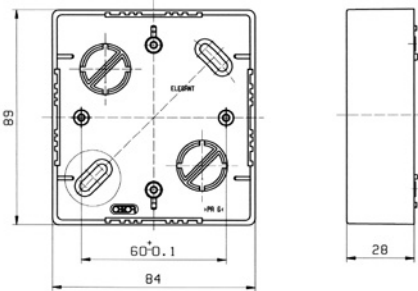
elektroinstalační krabice pro lištové rozvody
