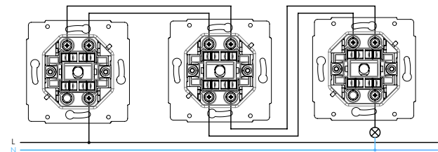
spínač řazení 6+7+6 střídavý - křížový - střídavý přepínač
