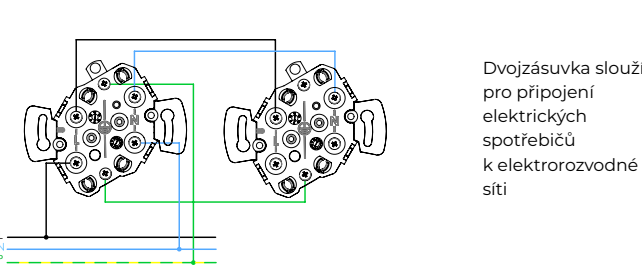
zásuvka dvojnásobná
