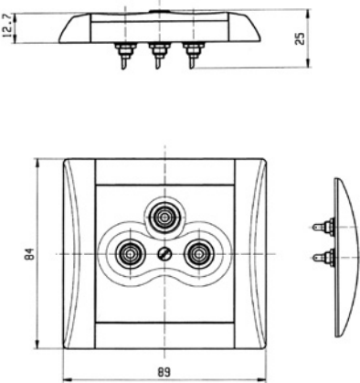
zásuvka AUDIO-VIDEO
