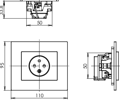
zásuvka jednonásobná s clonkou a zvukovou signalizací
