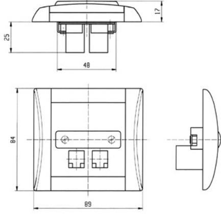
zásuvka komunikační
