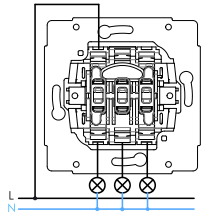
spínač řazení 1+1+1
