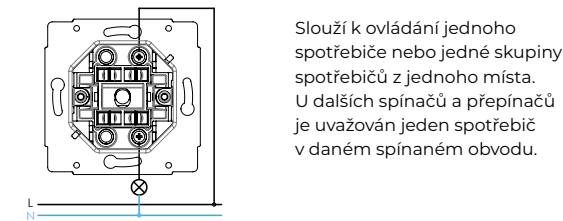
spínač řazení 1 (jednopolový vypínač)
